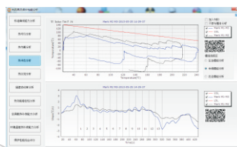
热冲击度
